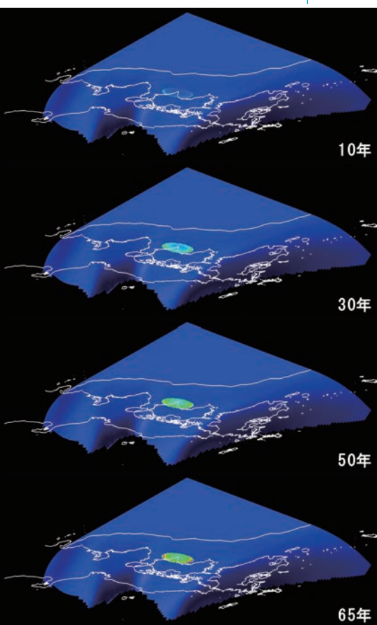
西南日本のプレート境界を対象とした 剪断応力蓄積シミュレーション
