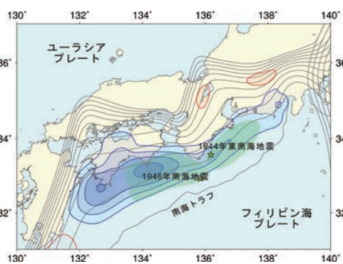
西南日本域のGPS変位速度データから推定したプレート間すべり遅れ速度分布。赤と青のコンターは、それぞれ、すべり過ぎとすべり遅れのプレートを表します。緑の領域は1944年東南海・1946年南海地震の津波波源域を表します。
