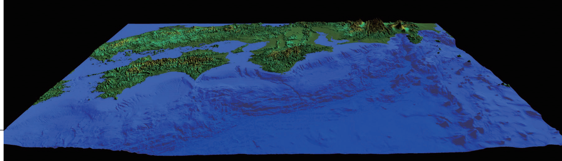
南海トラフ周辺の複雑な変動地形 (国土地理院、海上保安庁等の細密な標高データ から作成：広島大学他との共同研究成果)
